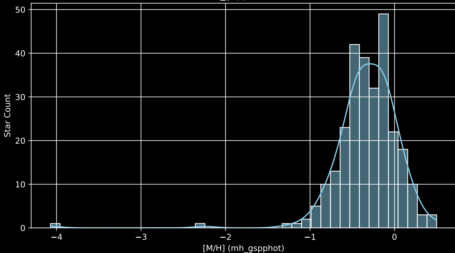
GALAH DR4 Field: [250] [M/H] (mh_gspphot) (n= 275)
