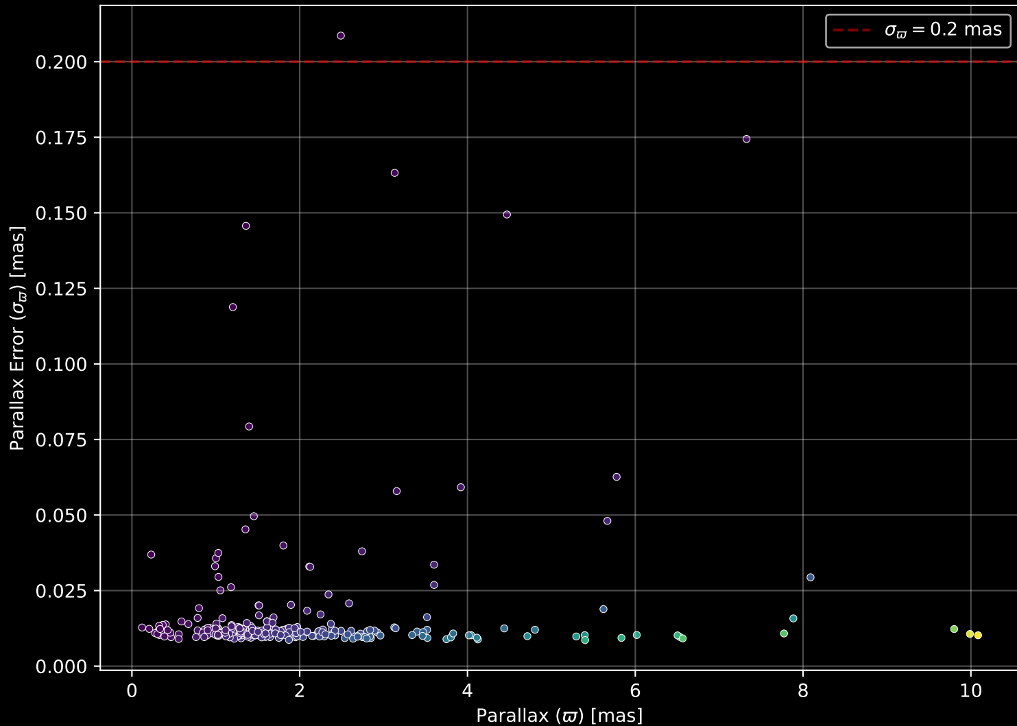
GALAH DR4 Field: [250] Parallax Quality (n= 278)
