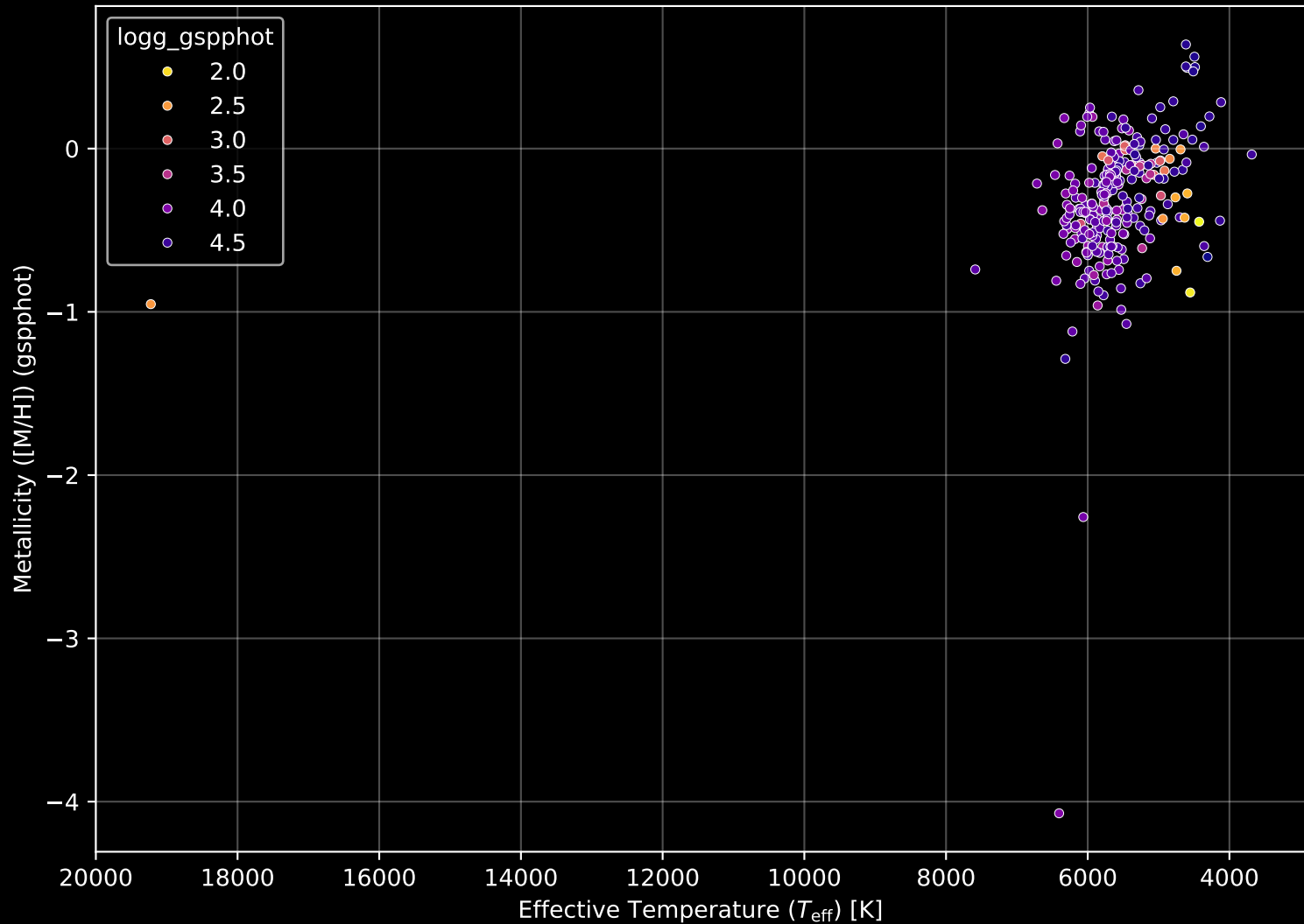
GALAH DR4 Field: [250] Stellar Population Parameters (n= 278)
