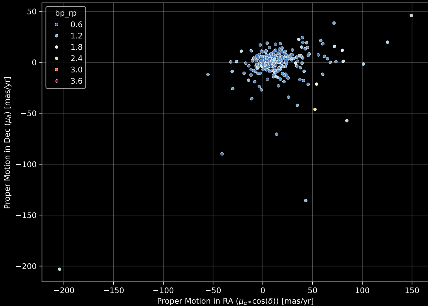
GALAH DR4 Field: [250] Proper Motion Diagram (n= 278)
